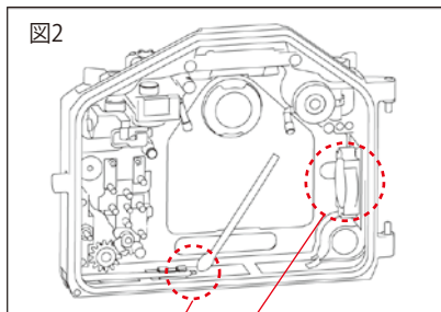
図2 リークセンサー端子 リークセンサー電池ボックス
